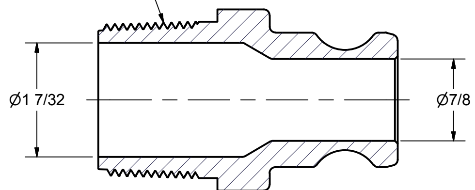
SECTION D-D SCALE 1 : 1
