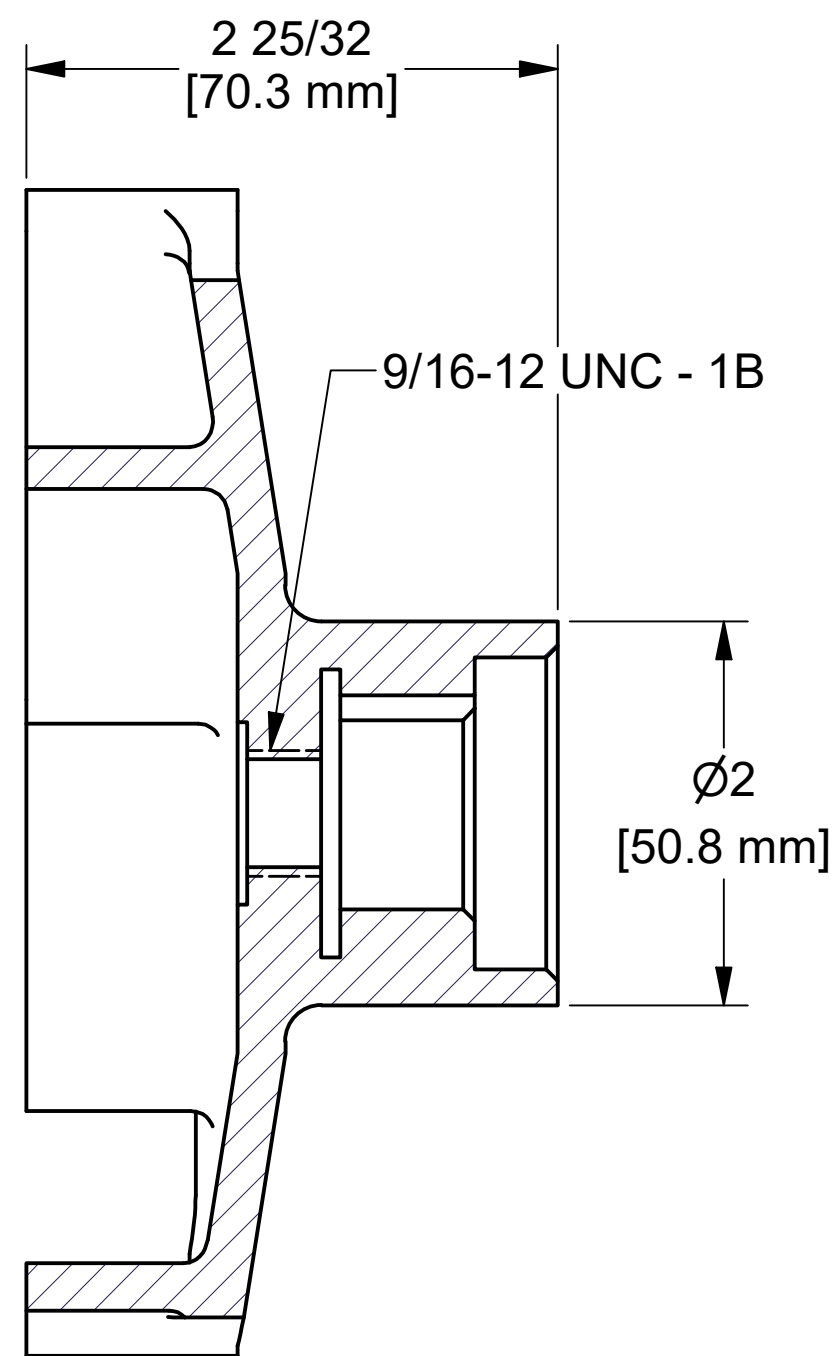
SECTION D-D SCALE 1 : 1
