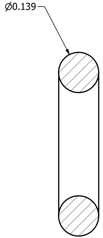
SECTION A-A SCALE 5 : 1
