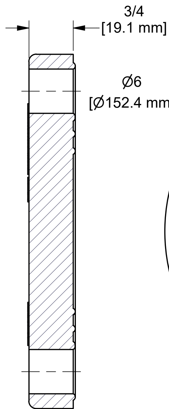
SECTION A-A SCALE 1 : 1
