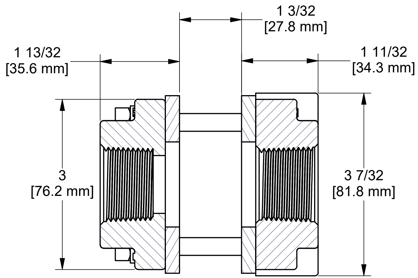
SECTION A-A SCALE 1 : 1
