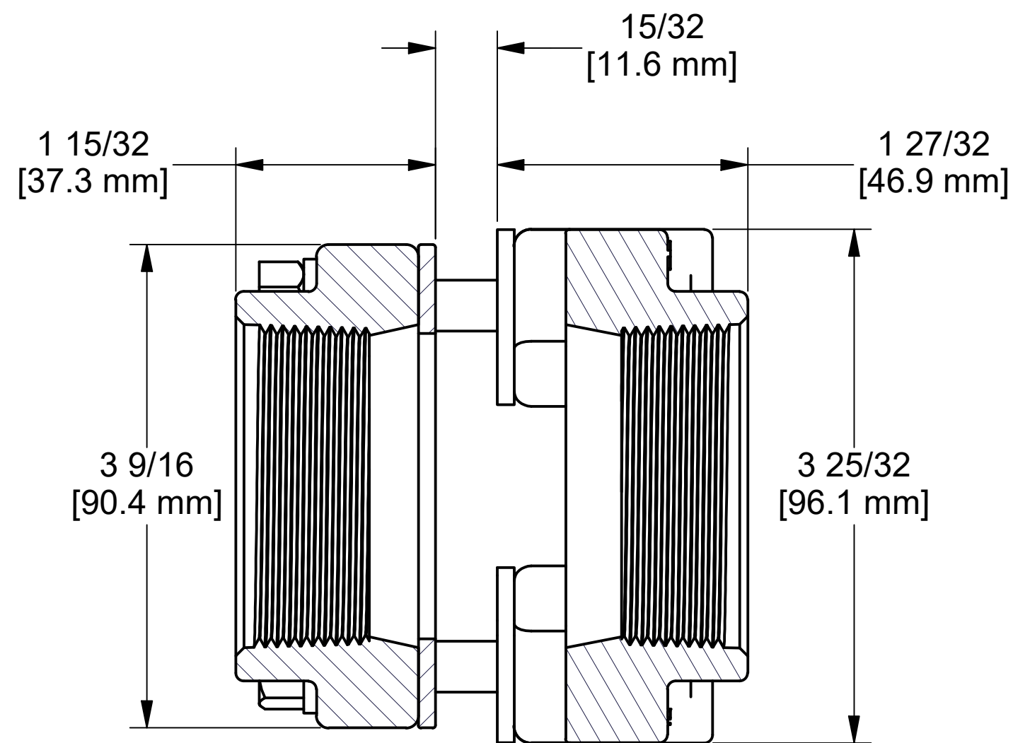
SECTION A-A SCALE 1 : 1
