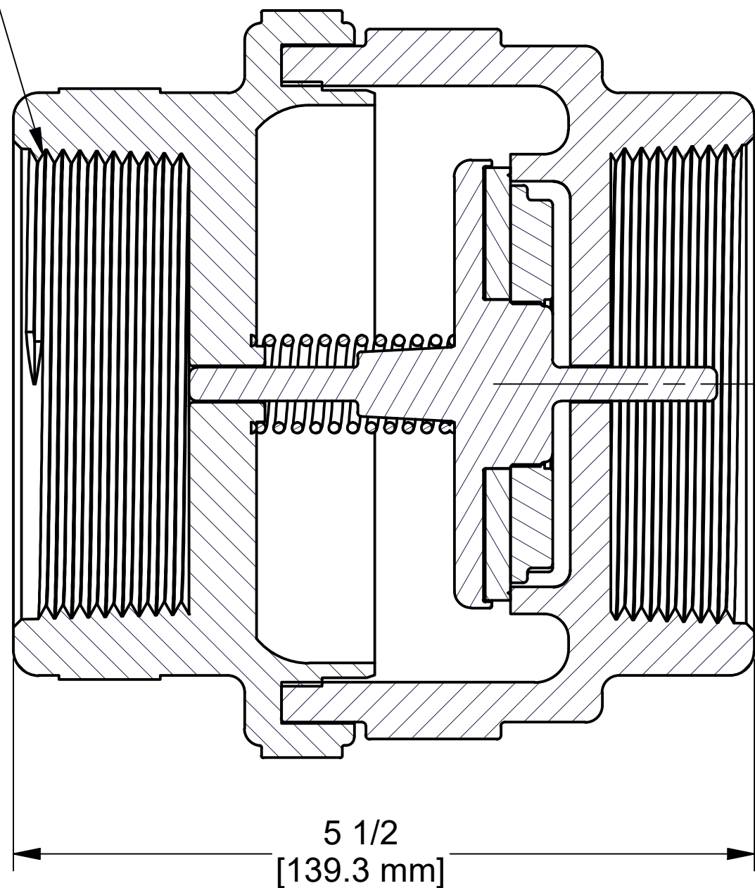
SECTION A-A SCALE 1 : 1
