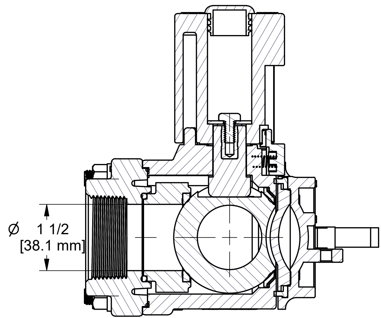
SECTION A-A SCALE 3 : 4
