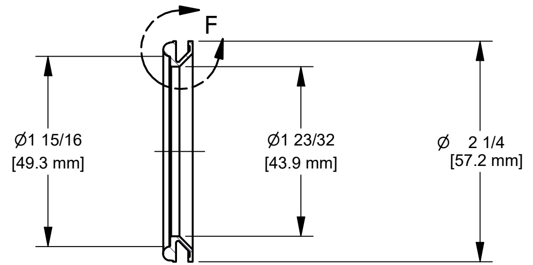
SECTION D-D SCALE 1 : 1
