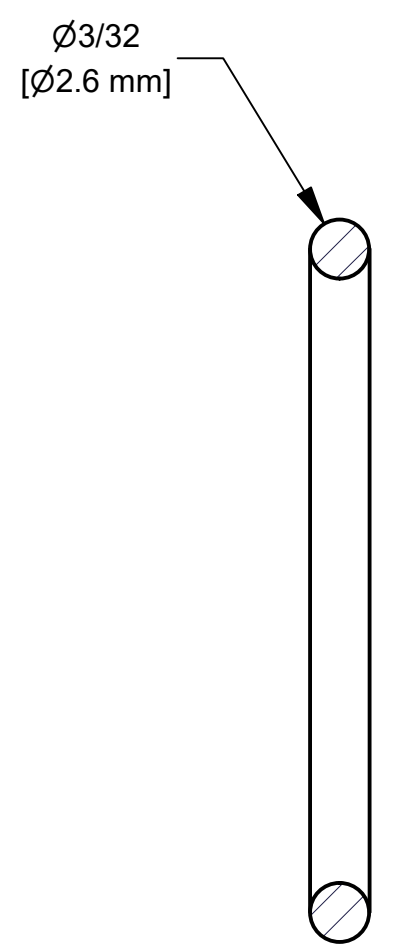
SECTION A-A SCALE 3 : 1
