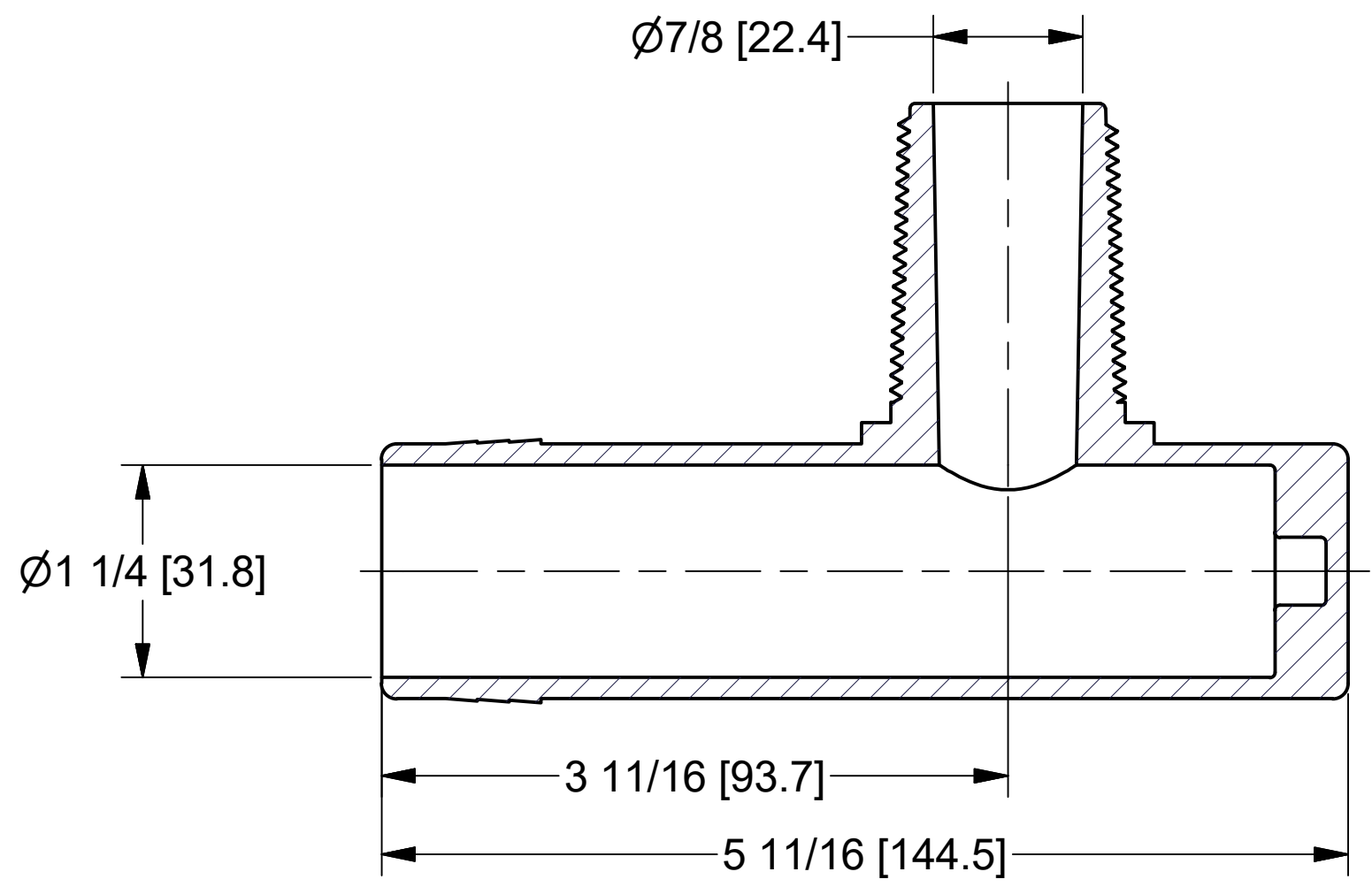
SECTION D-D SCALE 1 : 1
