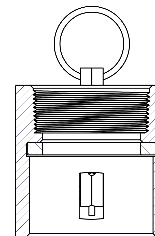
SECTION D-D SCALE 1 : 1
