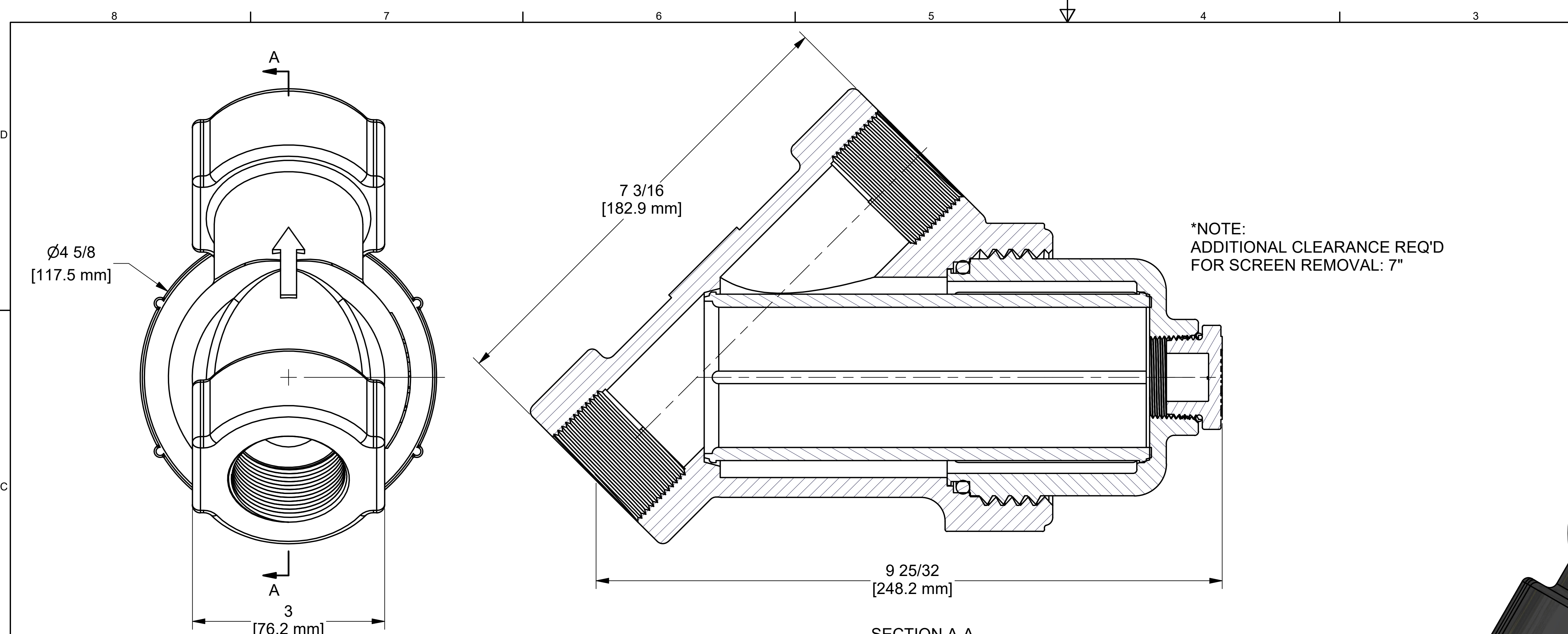
SECTION A-A SCALE 1 : 1
