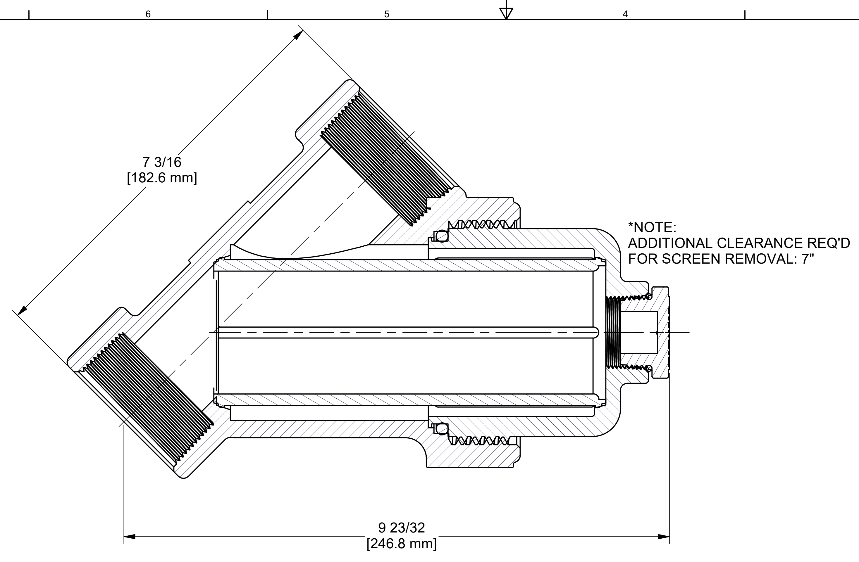
SECTION A-A SCALE 1 : 1
