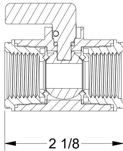
SECTION D-D SCALE 1 : 1
