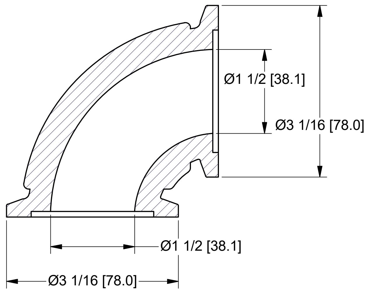
SECTION D-D SCALE 1 : 1
