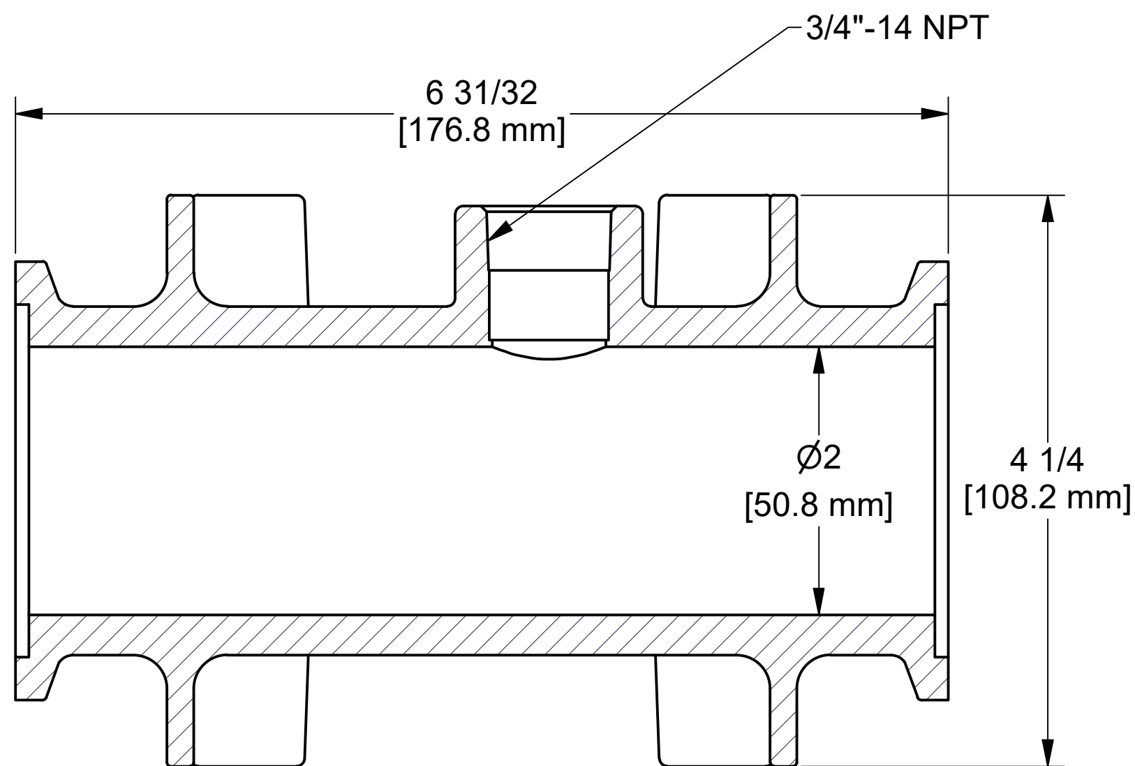
SECTION A-A SCALE 1 : 1
