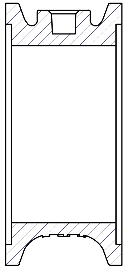
SECTION D-D SCALE 1 : 1
