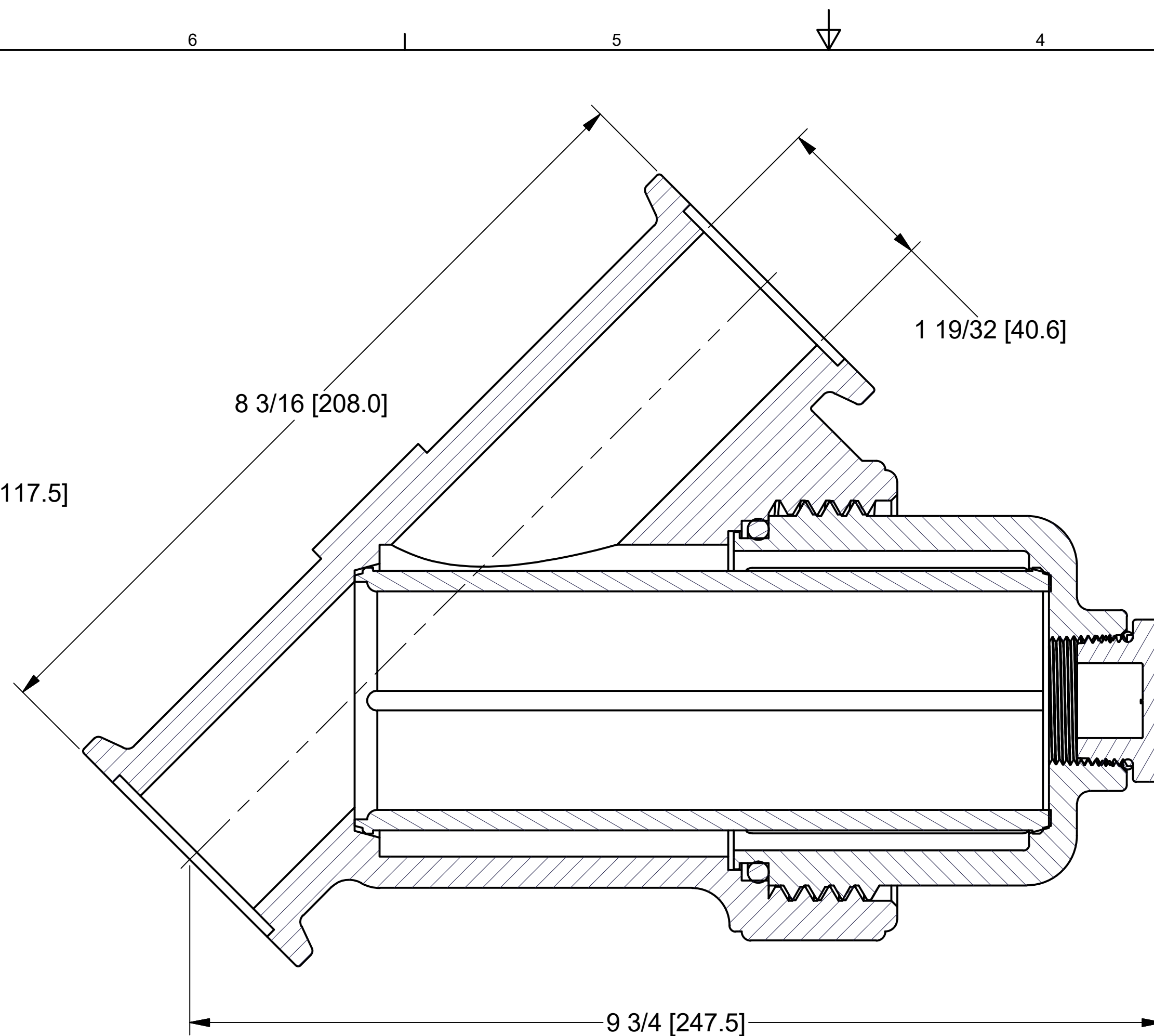
SECTION A-A SCALE 1 : 1
