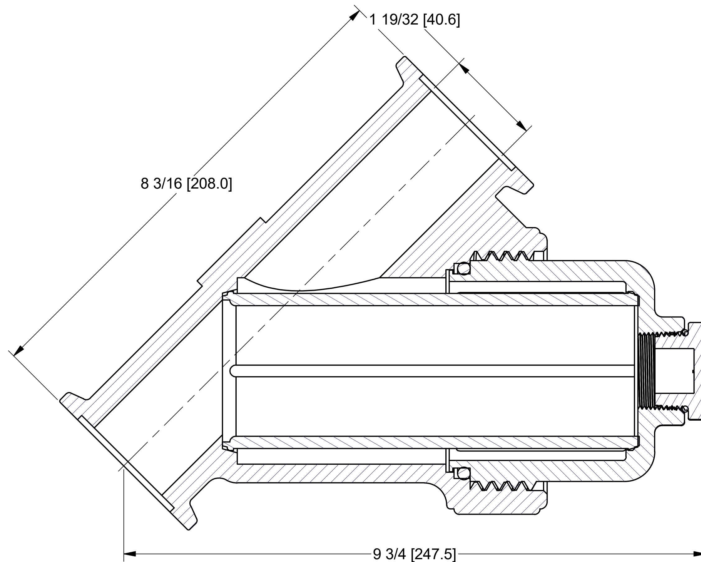
SECTION A-A SCALE 1 : 1
