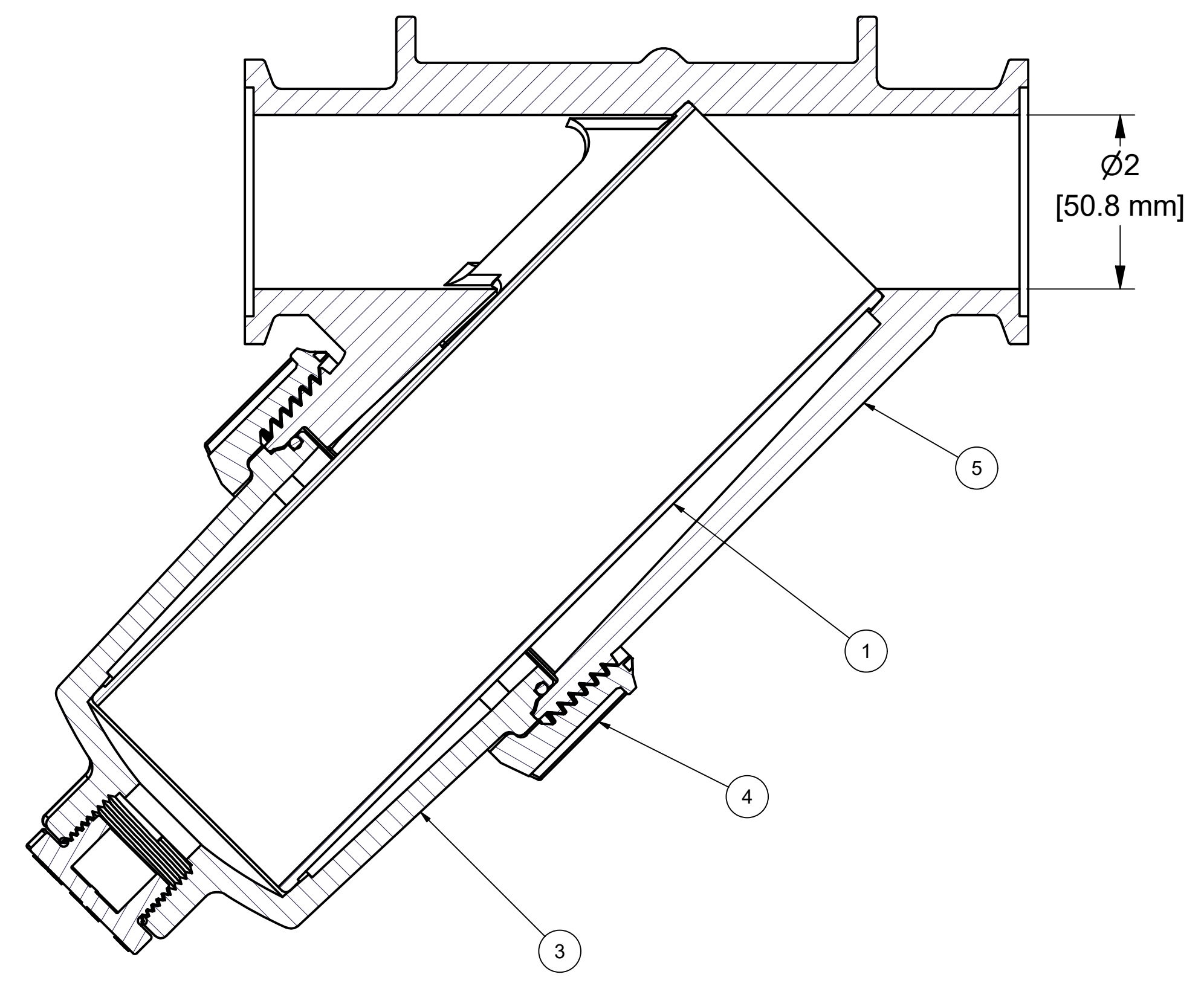
SECTION A-A
