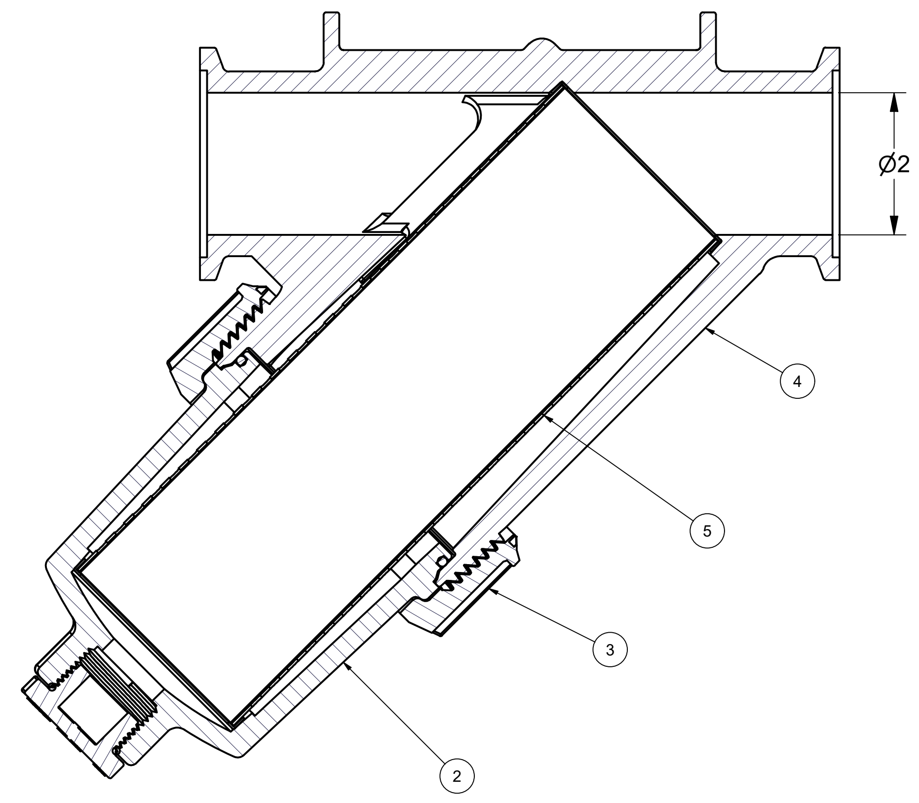
SECTION A-A
