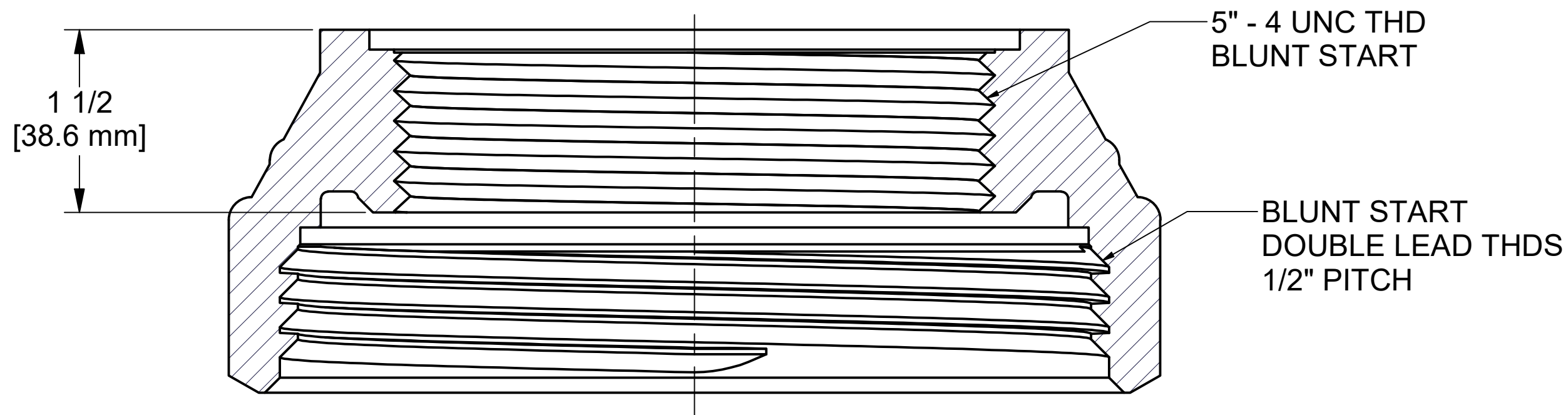
SECTION A-A SCALE 1 : 1
