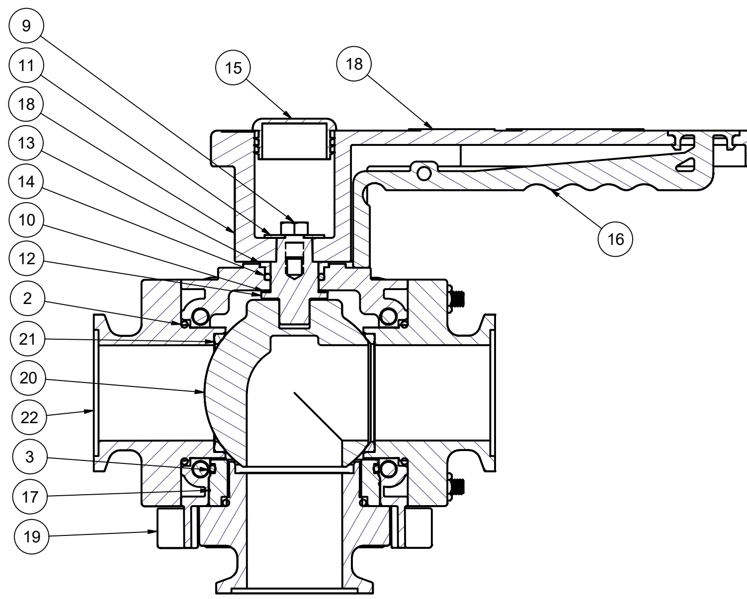
SECTION A-A
