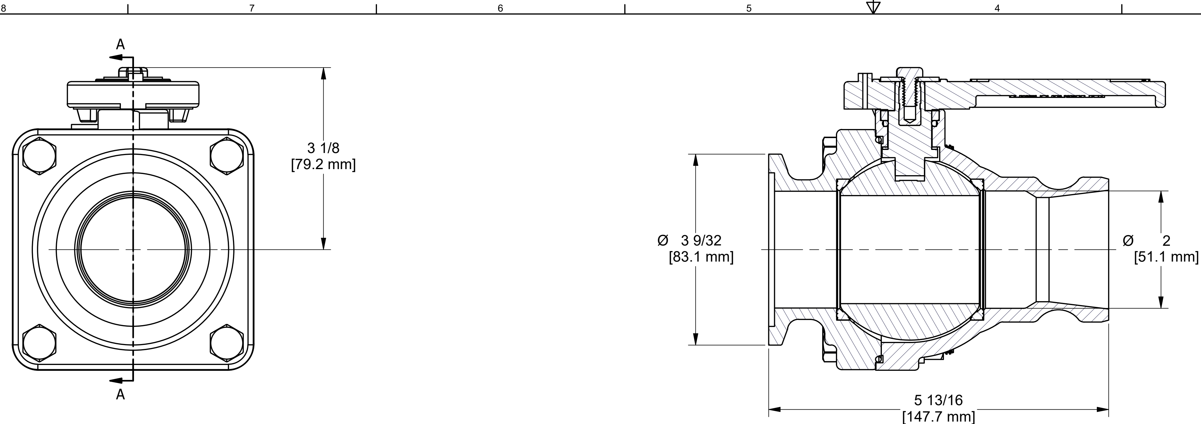
SECTION A-A SCALE 1 : 1
