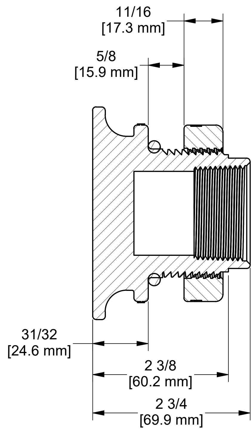
SECTION A-A SCALE 1 : 1
