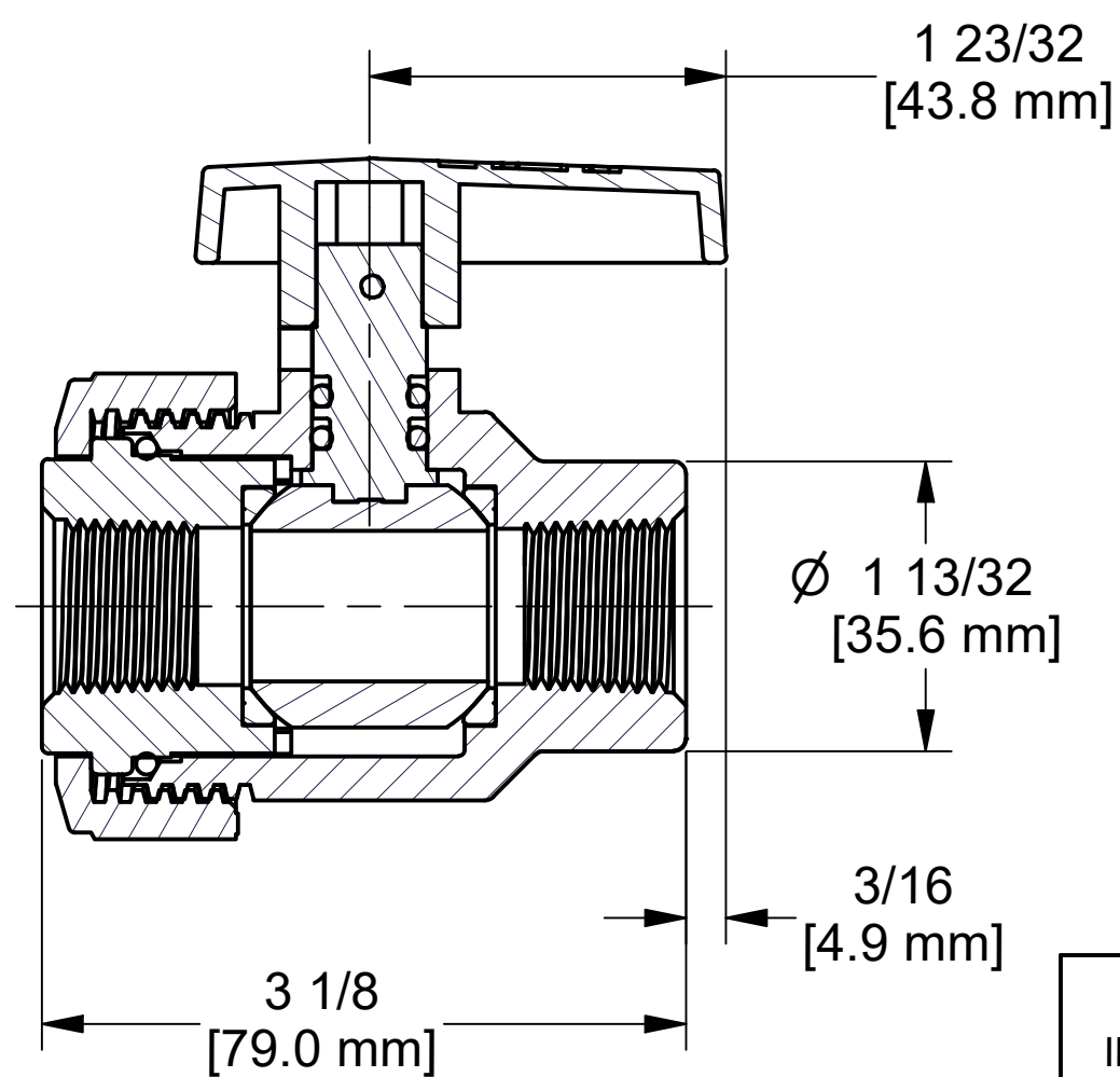
SECTION A-A SCALE 1 : 1
