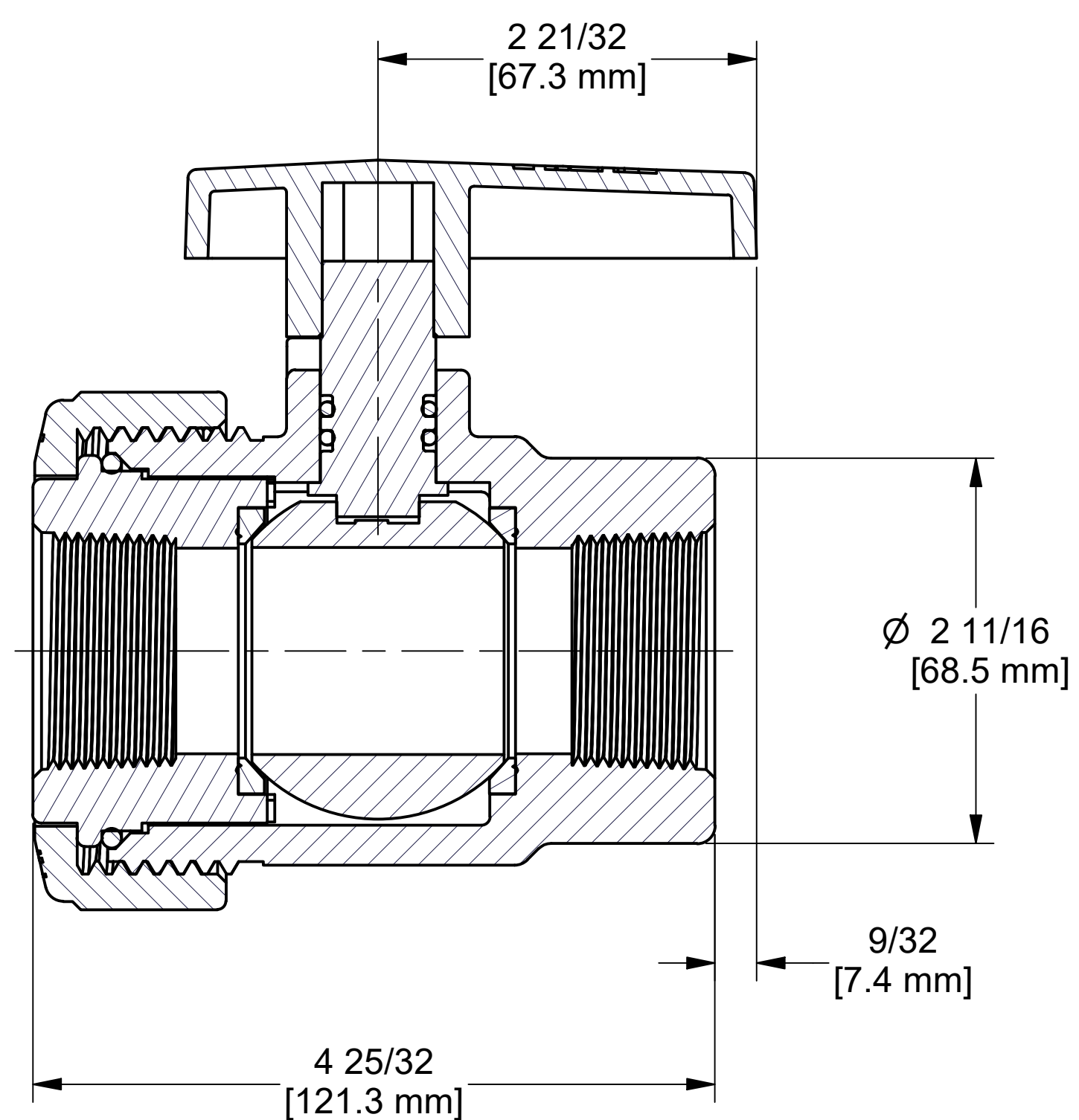
SECTION A-A SCALE 1:1
