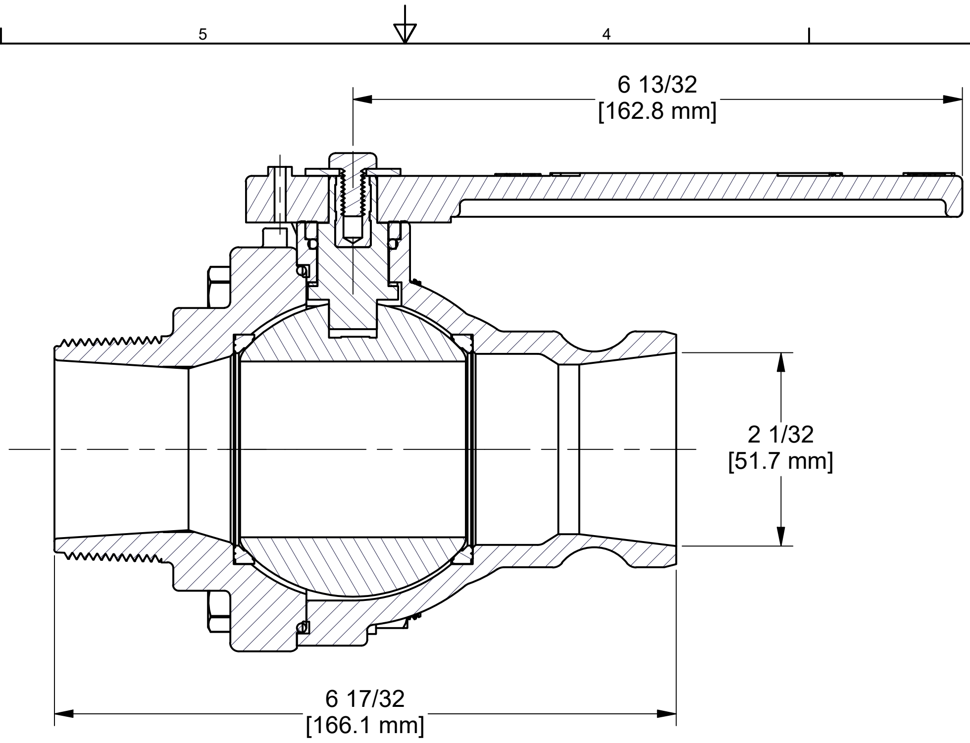
SECTION A-A SCALE 1 : 1
