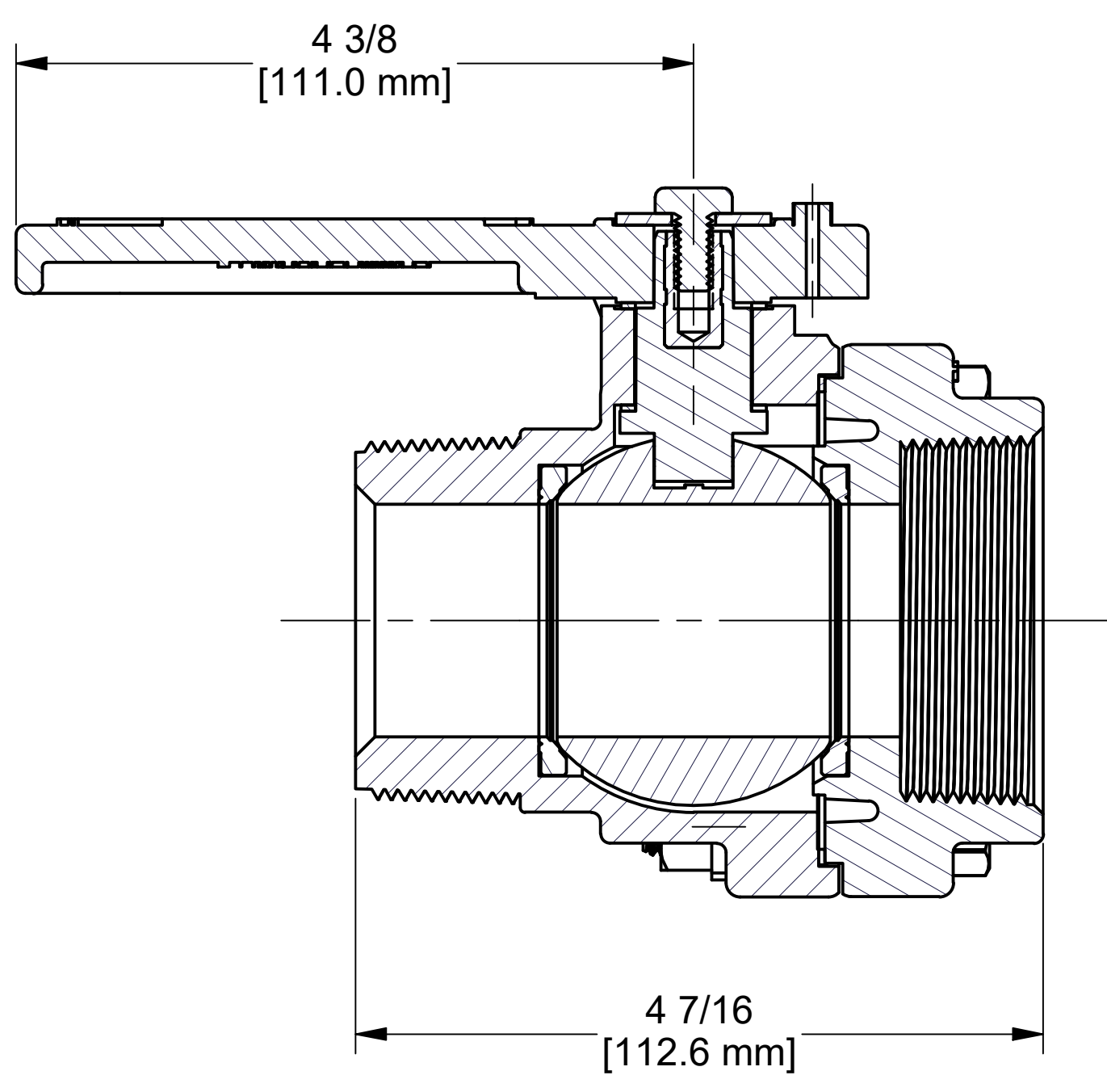
SECTION A-A SCALE 1 : 1
