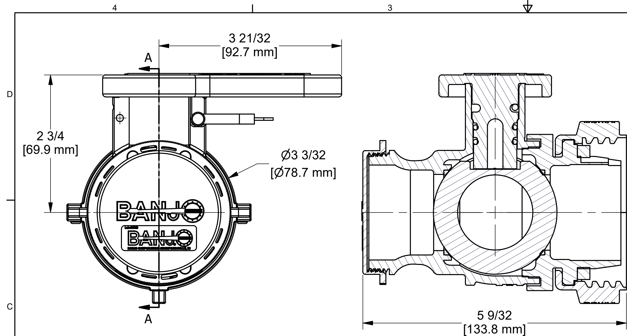
SECTION A-A SCALE 1 : 1
